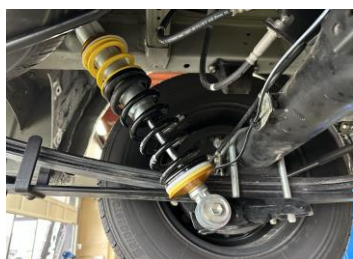
ロッド傷防止 スプリングカバー付き
