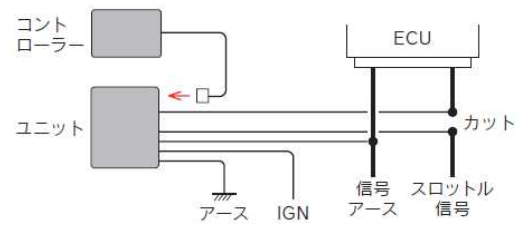
・コントローラー = 51 × 35 × 22mm (D) ・ユニット = 60 × 20 × 50mm (D)
